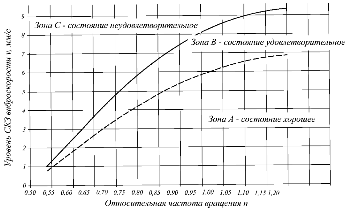
Рис. 9.9.3 Нормы вибрации винторулевых колонок
