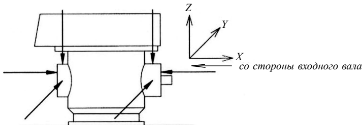
Рис. 9.9.2 Точки измерения вибрации винторулевых колонок
