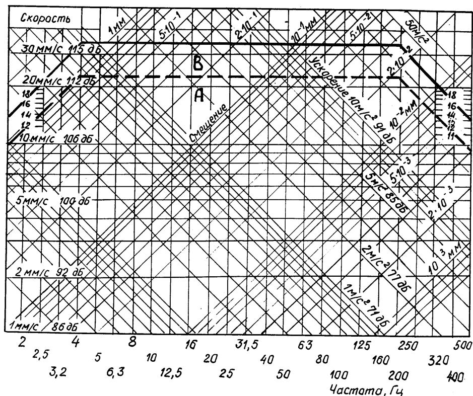
Рис. 9.3.4 Нормы вибрации турбокомпрессоров ДВС:
