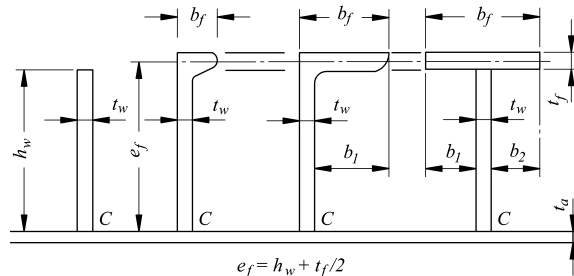
Рис. 7.10.6.31 Размеры ребра жесткости
