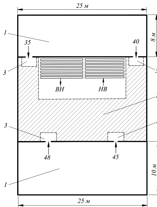
Рис. 7 Пример расчета загрузки общественных помещений:
