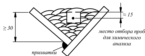
Рис. 4.9.2 Проба для испытаний наплавленного металла
