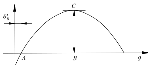
Рис. 1.3 Определение опрокидывающего момента в нерабочем состоянии
